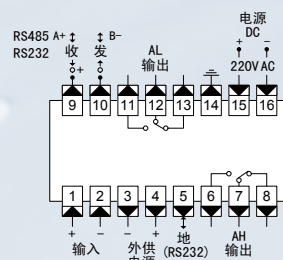
■ D规格96×48尺寸仪表
